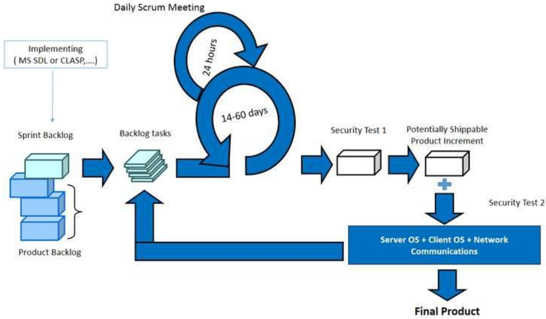
الشكل (6): إطار العمل الأمني لتطوير برامج Scrum
