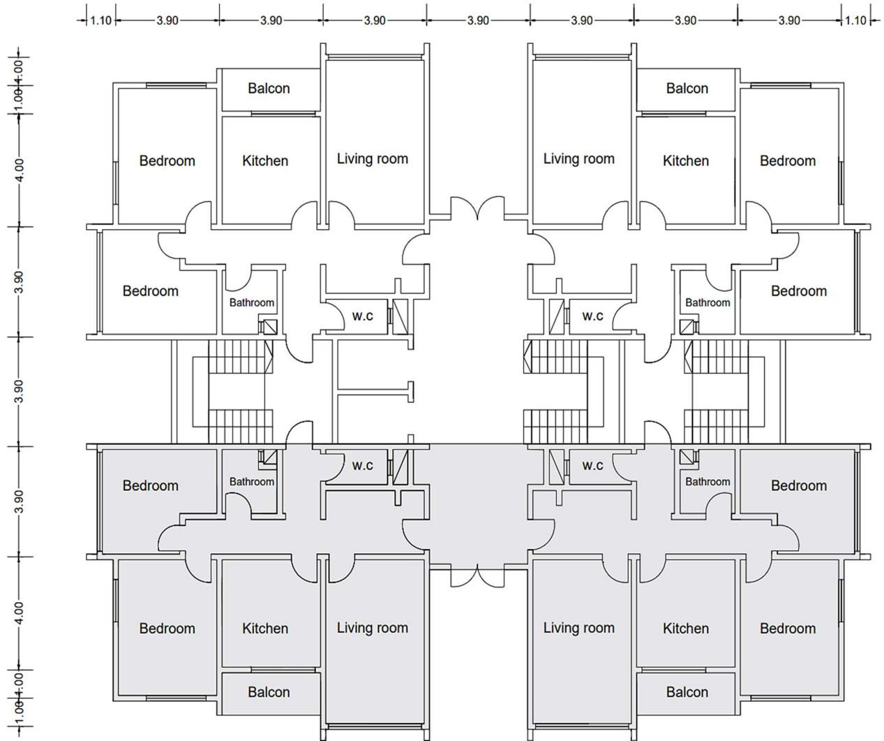
الشكل (1) مخطط الطابق للمبنى السكني
