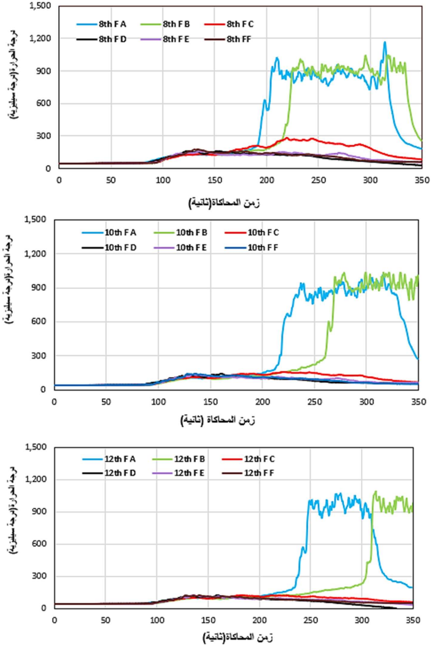
الشكل (10): تغير درجة الحرارة مع زمن المحاكاة عند الطوابق الثامن والعاشر والثاني عشر نماذج المساحة الفاصلة بين الشقق السكنية [A, B, C, D, E, F].
