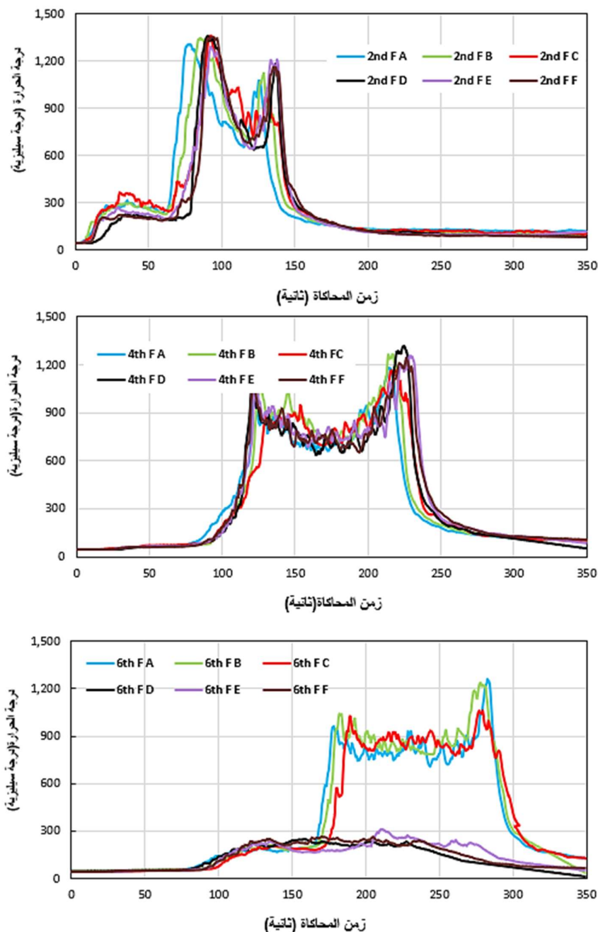
الشكل (9): تغير درجة الحرارة مع زمن المحاكاة عند الطوابق الثاني والرابع والسادس لنماذج المساحة الفاصلة بين الشقق السكنية [A, B, C, D, E, F].
